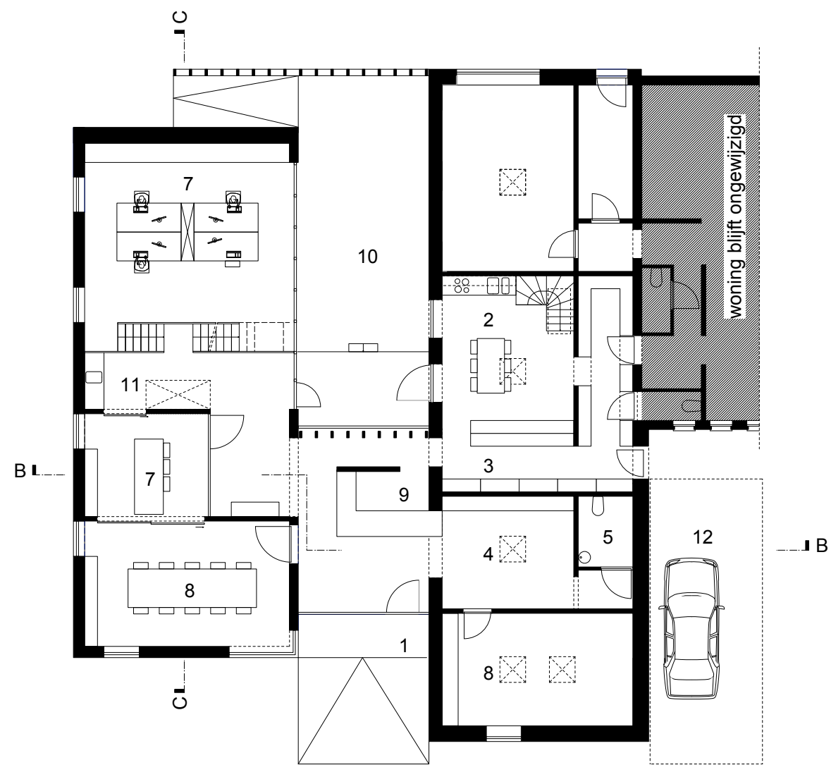
plan gelijkvloers
