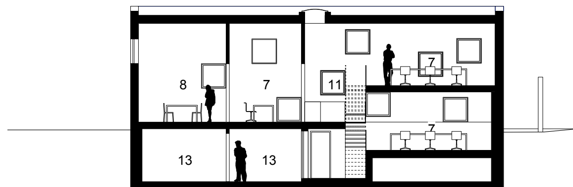
snede CC'
