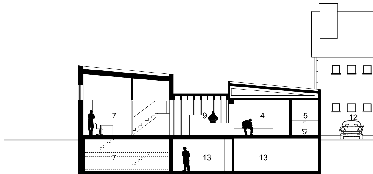
snede BB'
